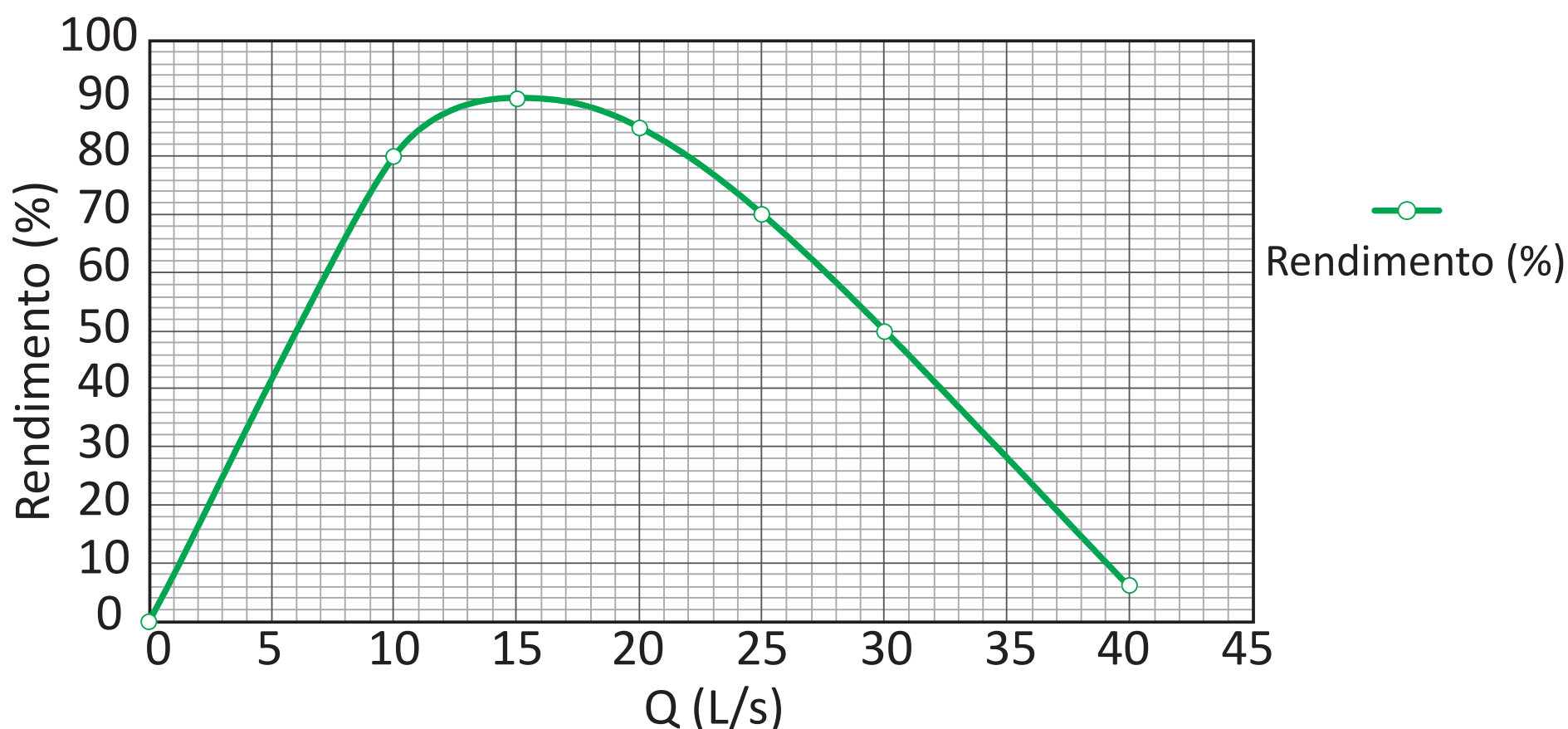
Figura 2 – Curva característica vazão versus rendimento
