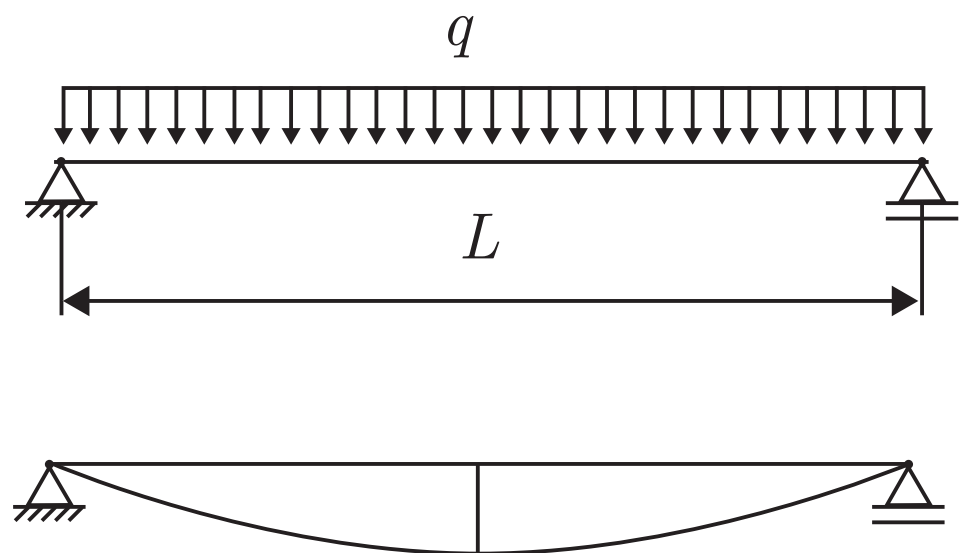
Carregamento e diagrama momento fletor - Viga
