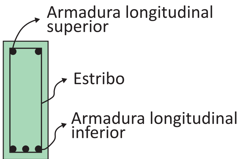
Seção transversal - Viga
