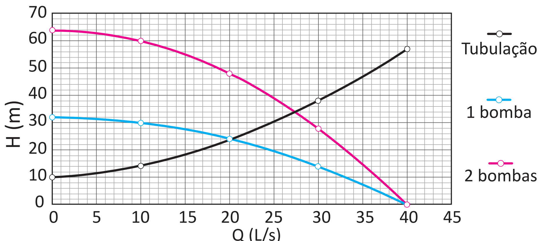
Figura 1 – Curvas características vazão versus altura manométrica
