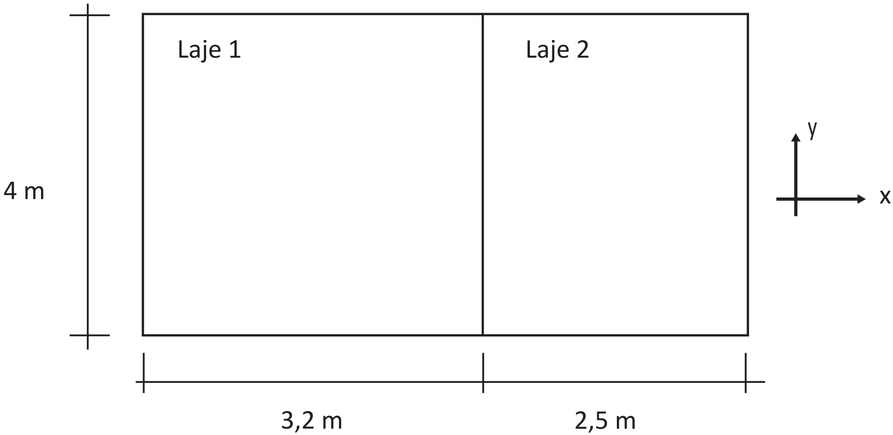
Figura 1 – Planta das lajes
